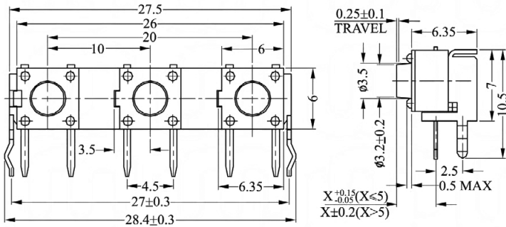
TCM-13AT ~ 13HZ
