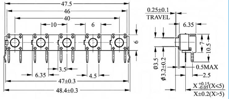
TCM-15AT ~ 15HZ
